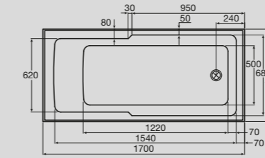
Domaine Shower Bath
